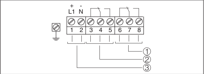
插图. 11: 单腔式外壳的接线图
