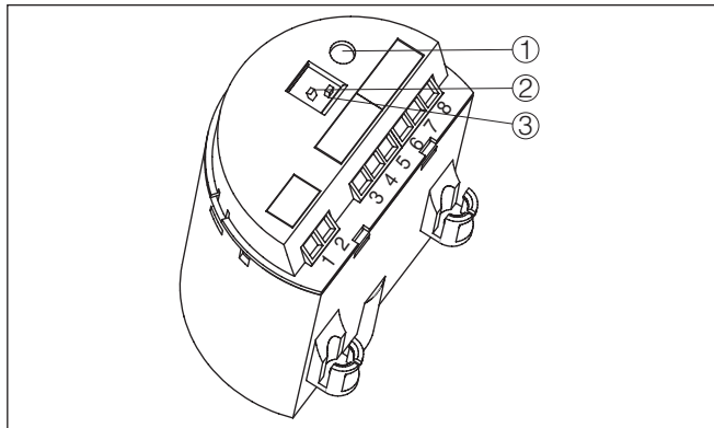
插图. 12: 电子插件 SWE60R - 继电器输出
