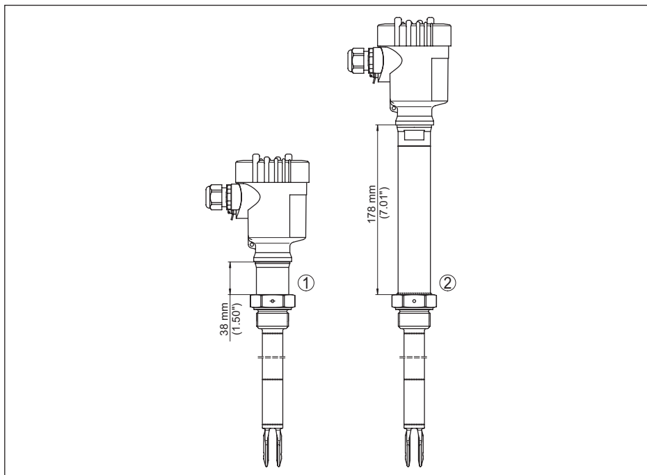
插图. 21: 选购件
