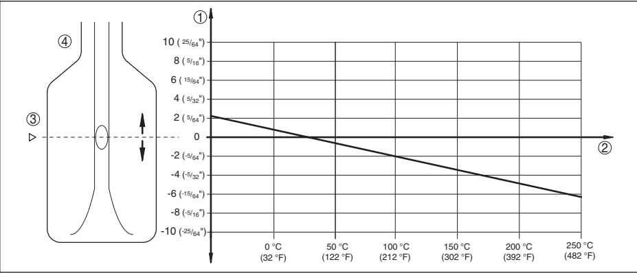
插图. 13: 过程温度对开关点的影响
