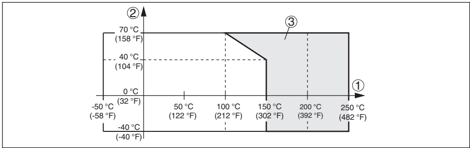
插图. 16: 环境温度 - 过程温度
