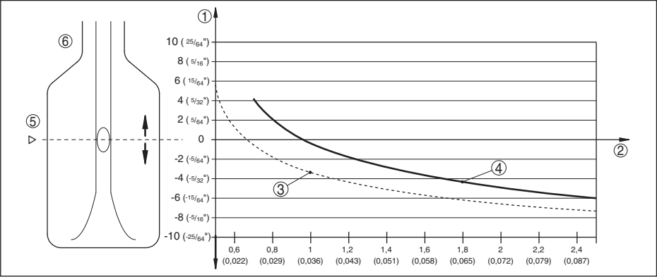
插图. 14: 介质密度对开关点的影响
