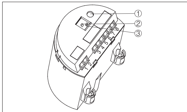
插图. 10: 电子插件 SWE60R - 继电器输出
