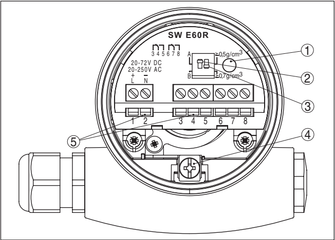
插图. 8: 电子部件和接线腔 单腔式壳体
