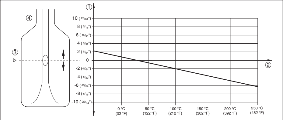
插图. 11: 过程温度对开关点的影响
