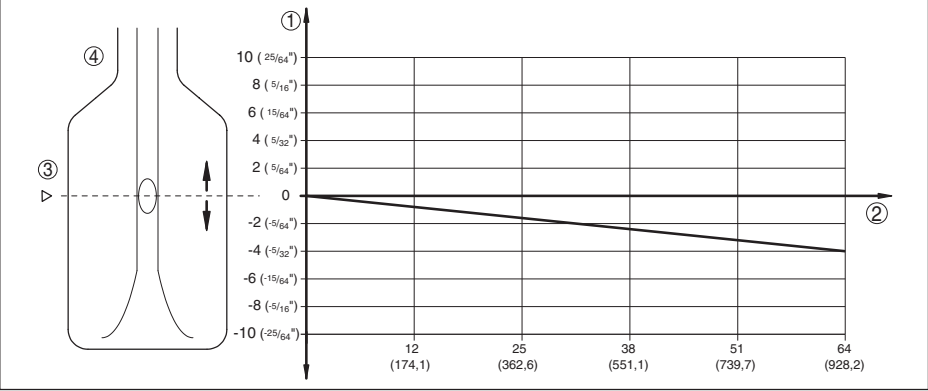
插图. 13: 过程压力对开关点的影响
