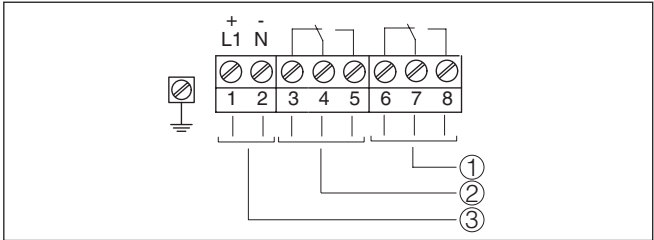
插图. 9: 单腔式外壳的接线图
