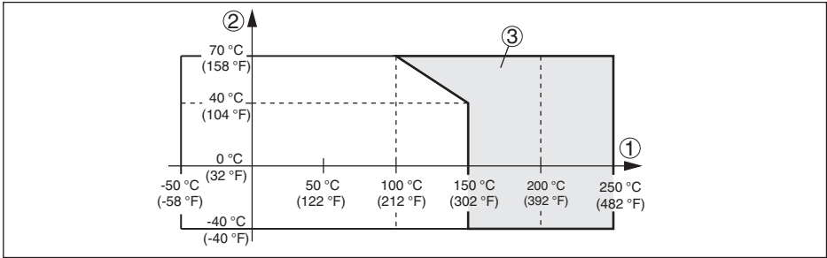
插图. 14: 环境温度 - 过程温度
