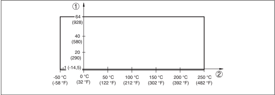
插图. 15: 过程温度 - 开关位置 \geq 0.7 \text{ g/cm}^3 时的过程压力 (灵敏度转换开关)
