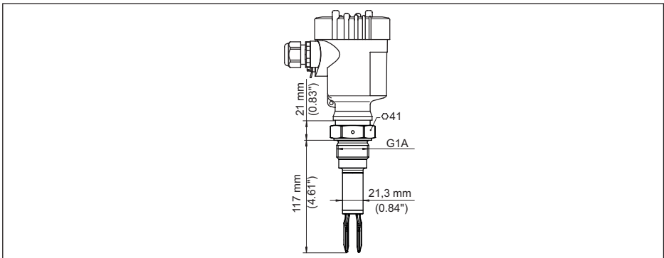
插图. 20: 开关位置延长件 - 用于方便更换 VEGASWING 81 或 81 A
