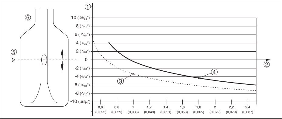
插图. 12: 介质密度对开关点的影响
