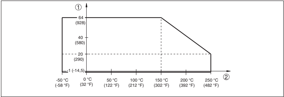
插图. 16: 过程温度 - 开关位置 \geq 0.5 \text{ g/cm}^3 时的过程压力 (灵敏度转换开关)
