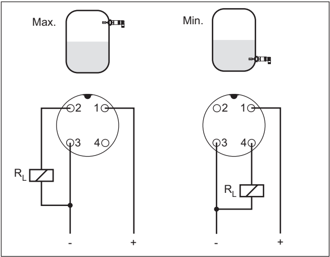
插图. 13: 接线图 (壳体)，采用 M12 x 1 插接头时的晶体管输出
