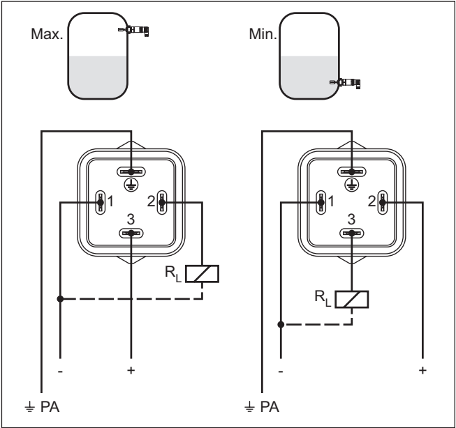
插图. 12: 接线图，阀塞 ISO 4400 的晶体管输出
