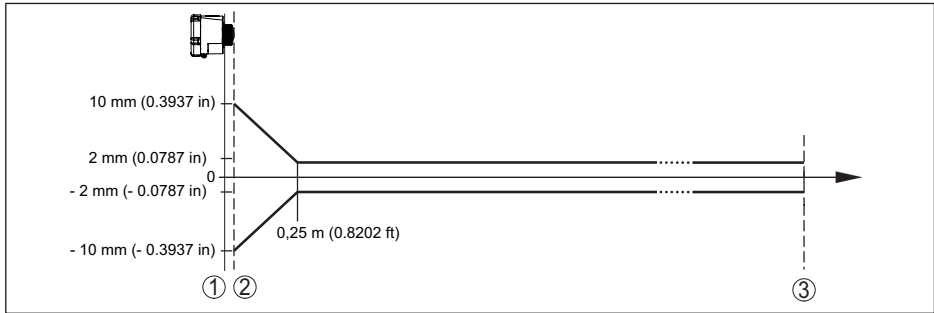
插图. 28: 在基准条件下的测量偏差
