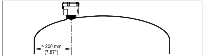
插图 5: 将雷达仪表安装在圆形容器盖上
