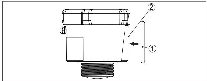
插图. 13: 激活仪表
