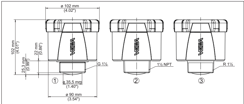
插图. 29: VEGAPULS Air 41 的尺寸
