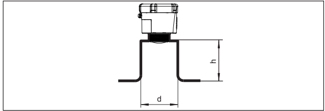
插图. 9: 当管接头的尺寸有别时管接头的安装
