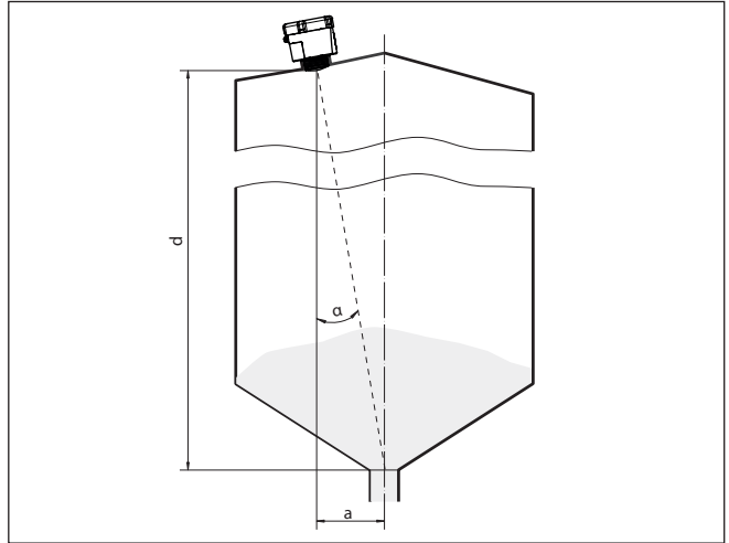
插图. 12: 校准 VEGAPULS Air 41 后的安装建议
