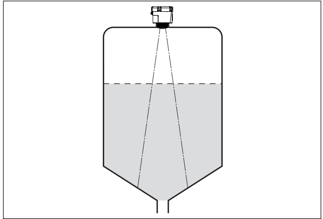
插图. 6: 将雷达仪表安装到带有锥形底部的容器上
