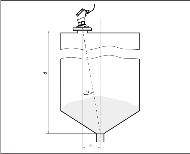
插图. 15: 校准 VEGAPULS 21 后的安装建议
