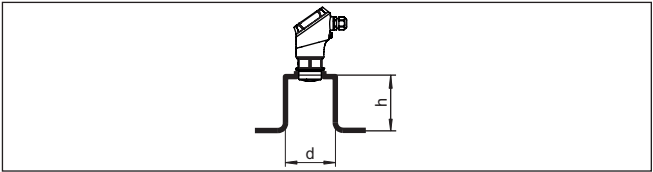
插图. 11: 管接头的安装
