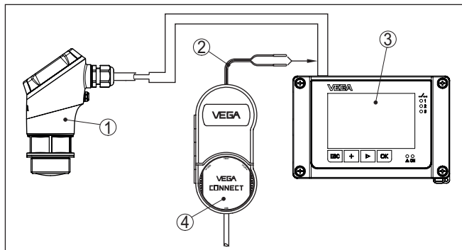
插图. 26: 将电脑与 VEGAMET 型控制器相连接
