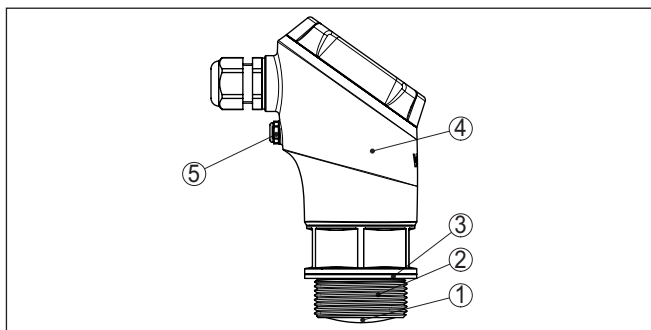
插图: 1: VEGAPULS 21的部件
