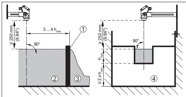
插图. 17: 用矩形槽测量流量： h_{\max} = 矩形槽的最大注水高度
