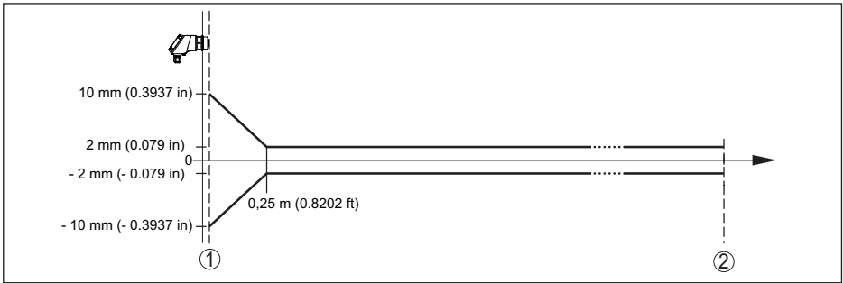
插图. 31: 在基准条件下的测量偏差 9)
