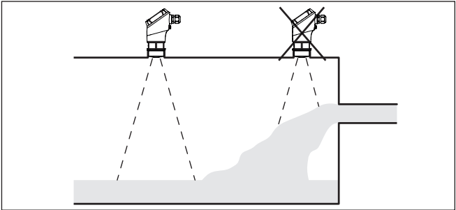
插图. 9: 流入介质时安装雷达传感器
