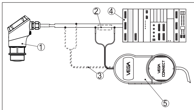
插图. 25: 将电脑与信号线路相连接
