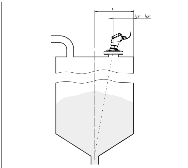
插图. 13: 安装位置和校准
