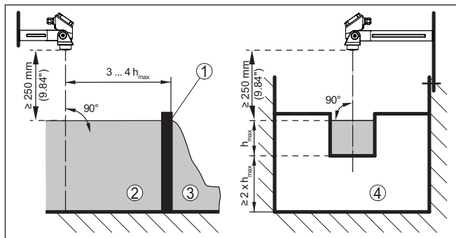
插图. 16: 用矩形槽测量流量： h_{\text{max}} = 矩形槽的最大注水高度
