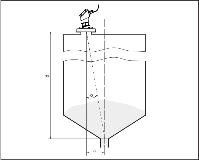
插图. 14: 校准 VEGAPULS 11 后的安装建议
