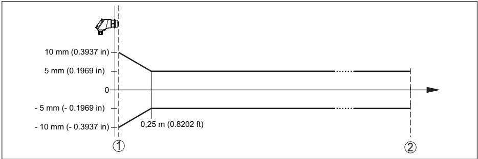
插图. 27: 在基准条件下的测量偏差 8)
