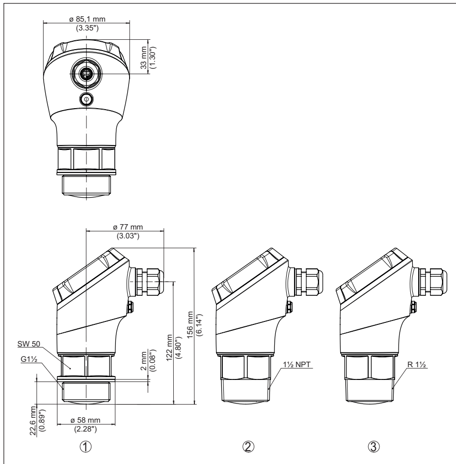
插图. 28: VEGAPULS 11 的尺寸
