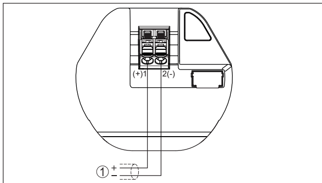
插图. 19: VEGAPULS 11 接线腔
