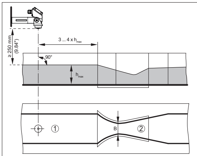
插图. 17: 用卡发基-文丘里槽来测量流量 : h_{\text{max}} =水槽的最大灌装量 ; B =水槽的最大收缩率
