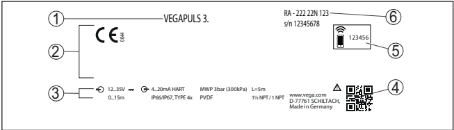
插图. 2: 铭牌的构造 (举例)
