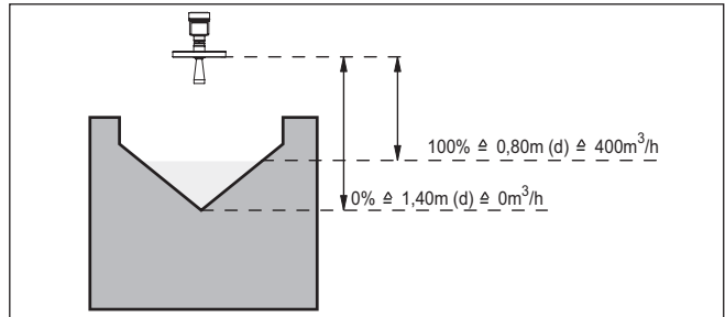
插图. 16: 用三角形水道调整流量的测量
