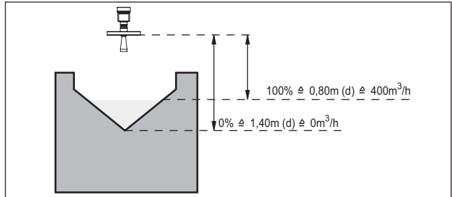
插图. 14: 用三角形水道调整流量的测量
