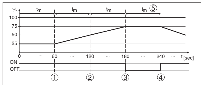
插图. 13: 趋势识别示例
