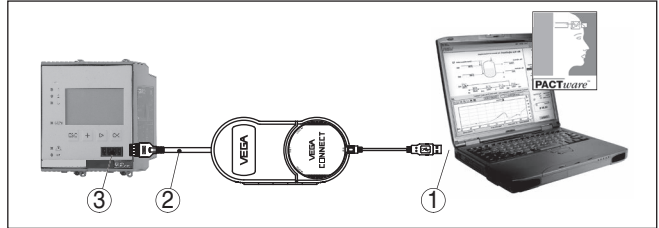
插图. 6: 通过 VEGACONNECT 进行连接
