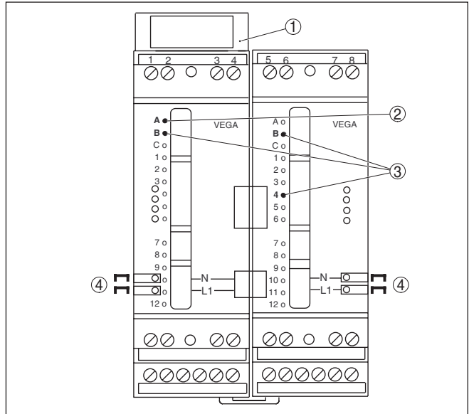
插图. 2: VEGAMET 624 的端子插座
