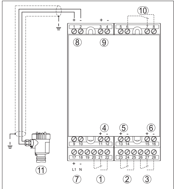
插图. 3: 带两线制传感器的接线图 VEGAMET 624
