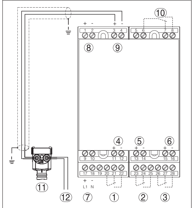
插图. 4: VEGAMET 624 与四线制传感器的接线图
