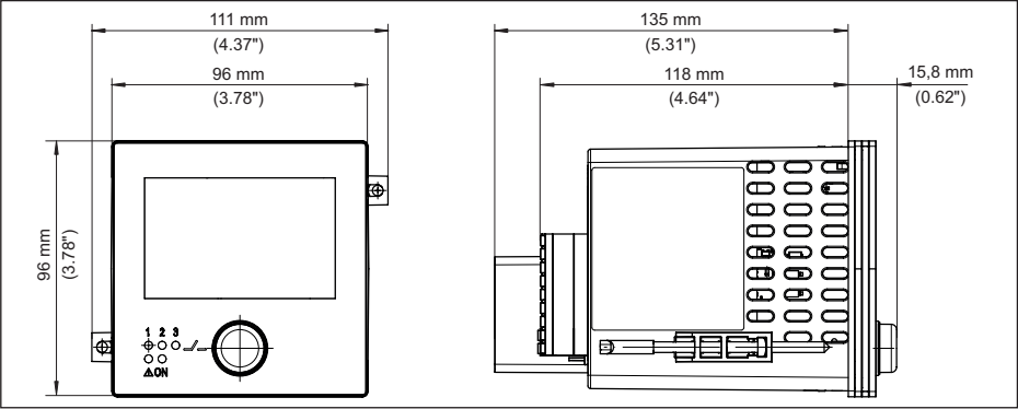
插图. 23: VEGAMET 342 的尺寸
