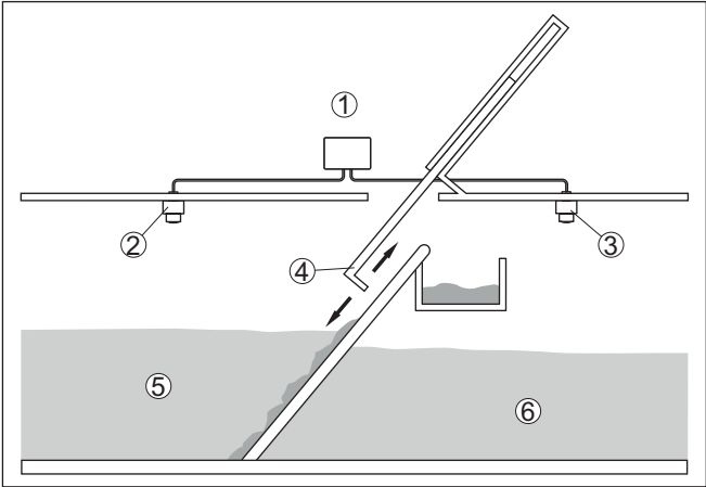
插图. 20: 格栅控制举例
