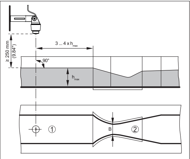
插图. 22: 用卡发基-文丘里槽来测量流量: h_{\text{max}} = 水槽的最大灌装量; B = 水槽的最大收缩率
