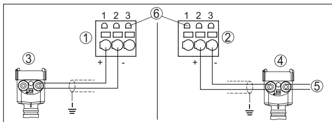
插图. 5: 输入接口 1, 用于两线制/四线制传感器 (有源/无源)
