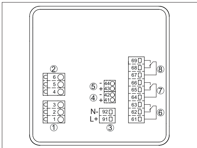
插图. 4: VEGAMET 342 的接线图
