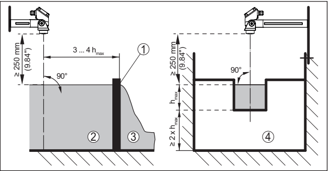
插图. 21: 用矩形槽测量流量: h_{\text{max}} = 矩形槽的最大注水高度
