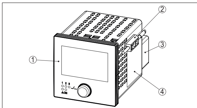
插图. 1: VEGAMET 342
