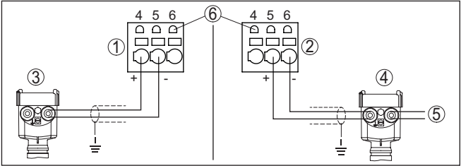
插图. 6: 输入端接口 2, 用于两线制/四线制传感器 (有源/无源)
