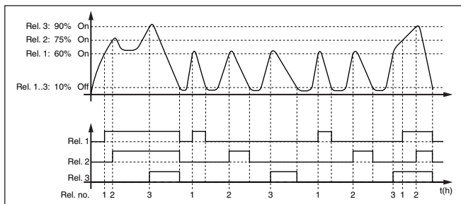
插图. 18: 泵控制器 4 的接通表现
