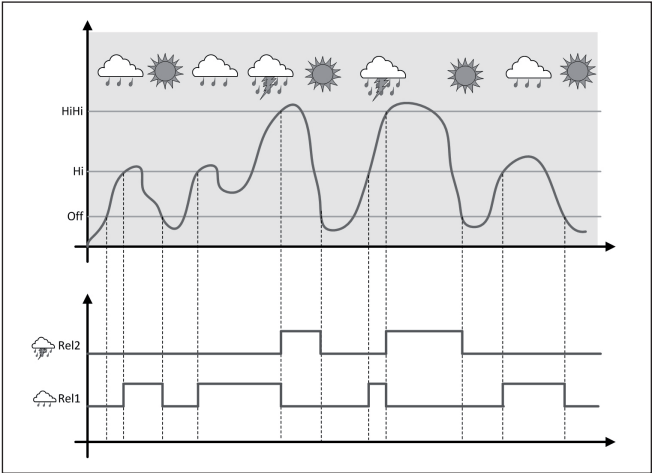
插图. 18: 用选项 "好天气运行" 来举例说明泵的控制
