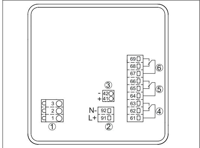
插图. 4: VEGAMET 341 的接线图
