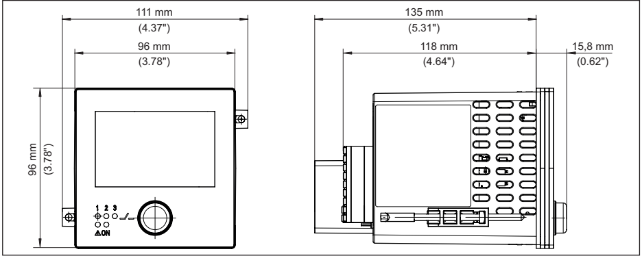
插图. 21: VEGAMET 341 的尺寸
