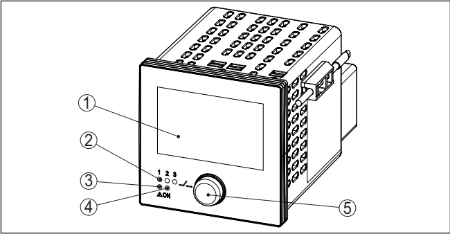
插图. 7: 显示和调整元件
