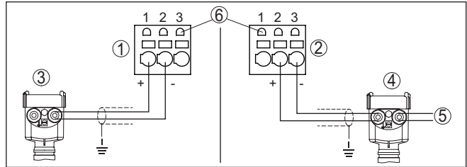
插图. 5: 输入接口 1, 用于两线制/四线制传感器 (有源/无源)
