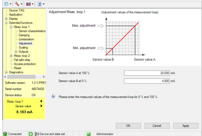
插图. 10: 一个 DTM 视图举例 - 调整
