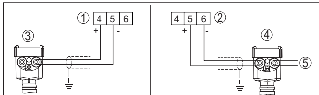
插图 5: 传感器输入端 2 的接口, 用于两线制/四线制传感器 (有源/无源)
