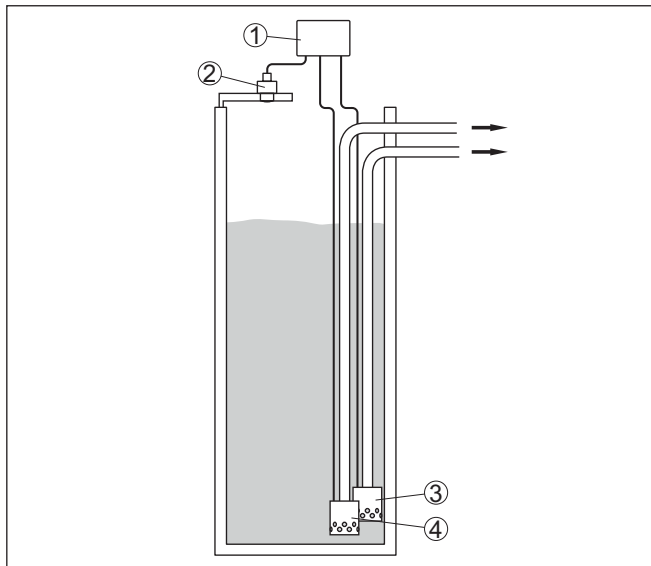
插图. 12: 泵站举例：在流入沟口控制泵
