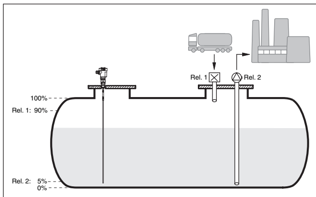
插图. 11: 举例说明对卧式圆形槽罐的物位测量
