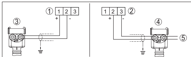
插图 4: 传感器输入端的接口, 用于两线制/四线制传感器 (有源/无源)
