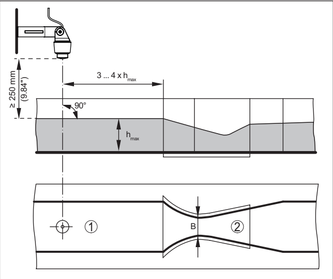
插图. 20: 用卡发基-文丘里槽来测量流量: h_{\text{max}} = 水槽的最大灌装量; B = 水槽的最大收缩率
