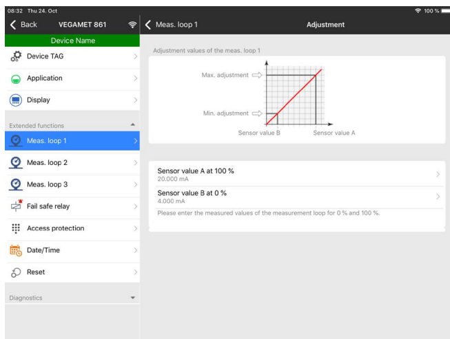
插图. 9: App 应用程序视图举例 - 调试 调整
