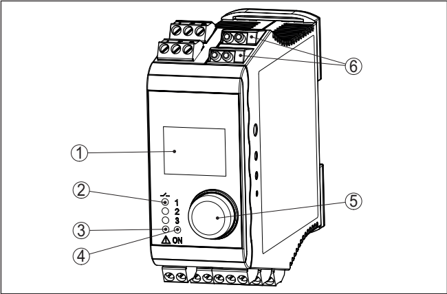
插图. 6: 显示和调整元件
