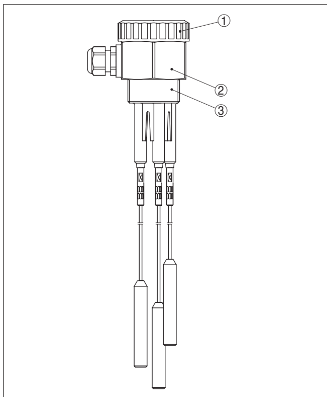
插图. 1: 导电性多缆式测量探头 EL 6
