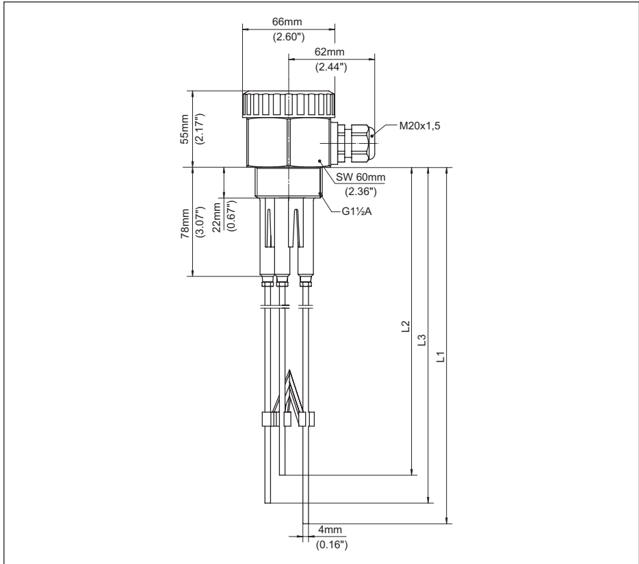
插图. 7: 导电性多棒式测量探头 EL 4
