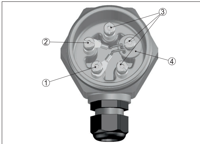
插图. 6: 请为电线断裂监控安装附加电子部件
