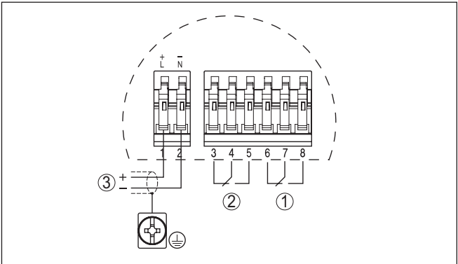
插图. 11: 接线图
