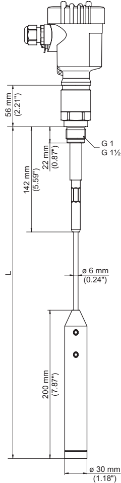
插图. 20: VEGACAP 65, 绳型 \varnothing 6 \text{ mm} (0.236 in), 螺纹型 G1 (ISO 228 T1)
