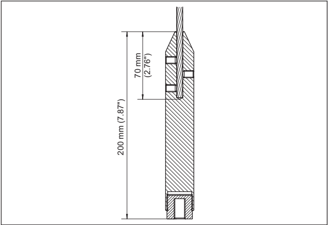
插图. 16: 兼顾重锤并相应地剪短绳缆
