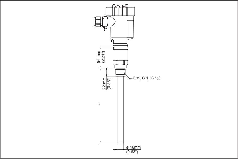
插图. 17: VEGACAP 63, 螺纹型 G1 (ISO 228 T1)
