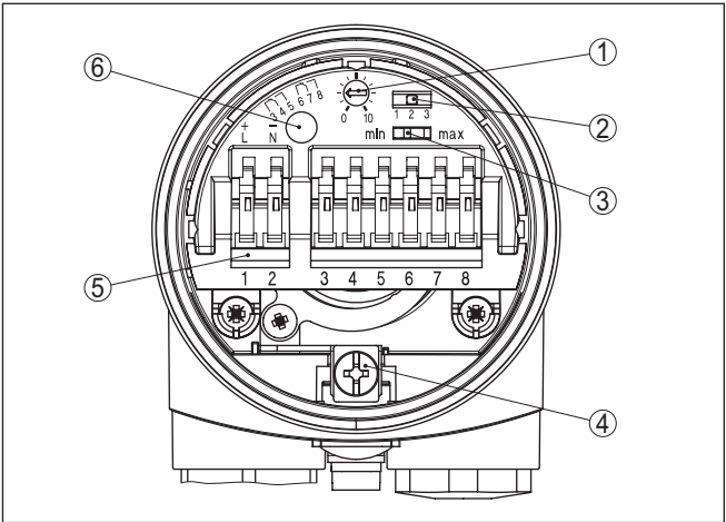
插图. 13: 带继电器输出电子插件
