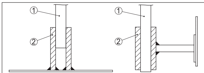
插图. 6: 将测量探头固定好
