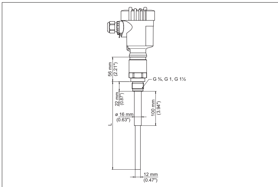
插图. 34: VEGACAL 62, 螺纹型 G1 (ISO 228 T1)
