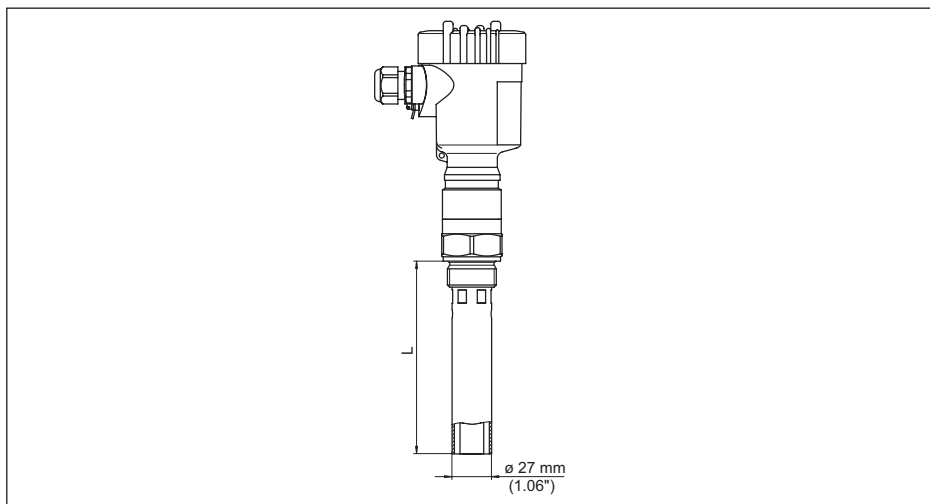
插图. 37: VEGACAL 62, 封管, 比如在介电常数较小时或进行线性化时
