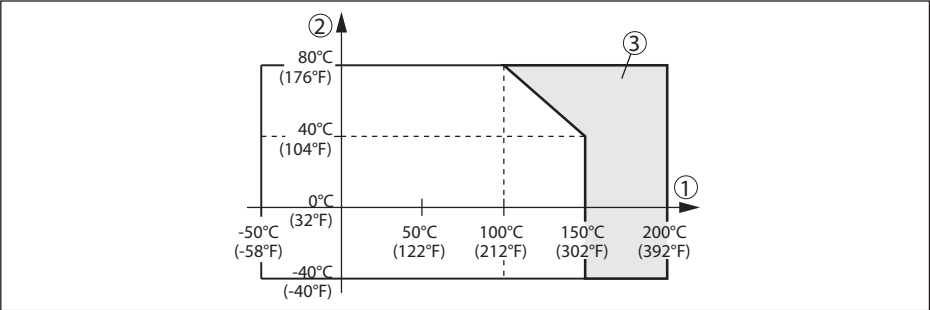
插图. 30: 环境温度 - 过程温度
