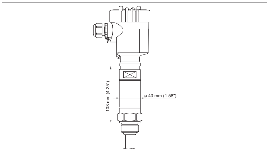
插图. 35: 温度连接元件
