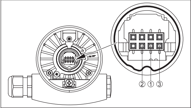
插图. 28: 检查测量探头内的电阻
