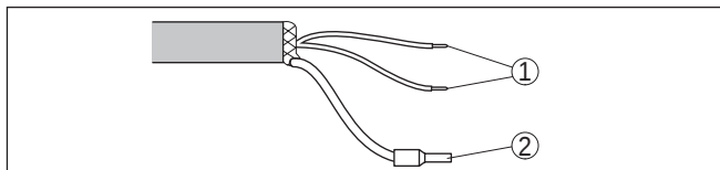
插图. 19: 连接电缆的芯线分布
