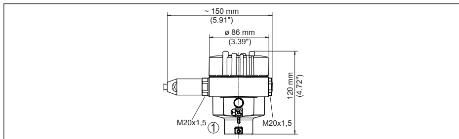
插图. 33: 采用防护等级达 IP66/IP68 (1 bar) 的壳体版本 (内装显示和调整模块后, 壳体高度增加了18 mm/0.71 in)
