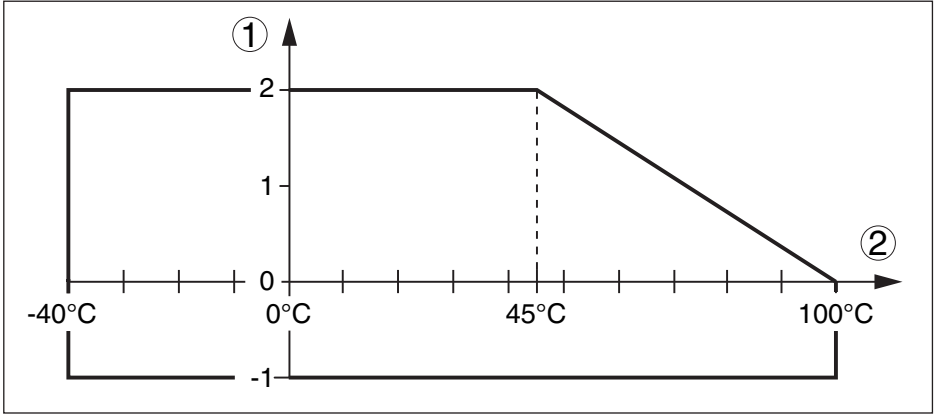
插图. 29: 过程压力 - 过程温度 (用 PTFE 制成的法兰)
