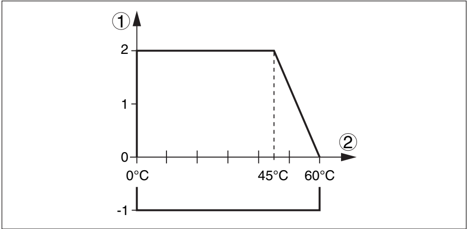
插图. 30: 过程压力 - 过程温度 (用 PP 制成的法兰)
