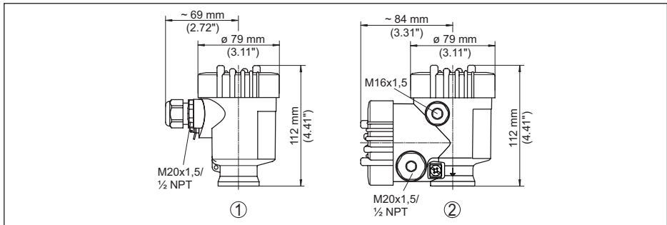
插图: 32: 采用防护等级为 IP66/IP67 的外壳版本 (内装显示和调整模块后，外壳高度增加了 9 mm/0.35 in)
