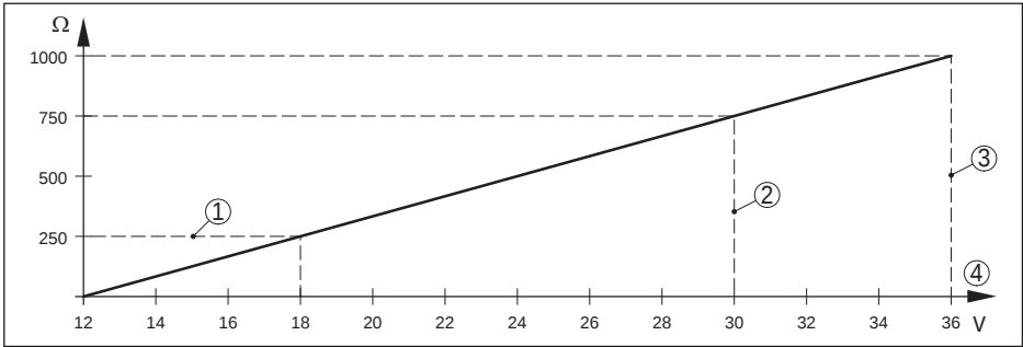
插图. 31: 供电电压图
