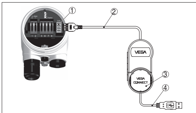
插图. 23: 通过接口适配器 VEGACONNECT 与外部相连
