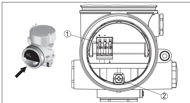
插图. 17: 防爆 (d ia) 型双腔式外壳的接线腔
