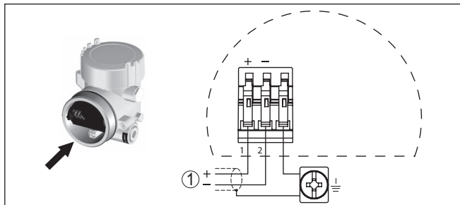
插图. 18: 防爆 (d ia) 型双腔式外壳的接线图
