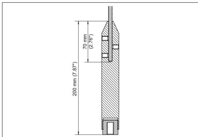
插图. 30: 兼顾重锤并相应地剪短绳缆
