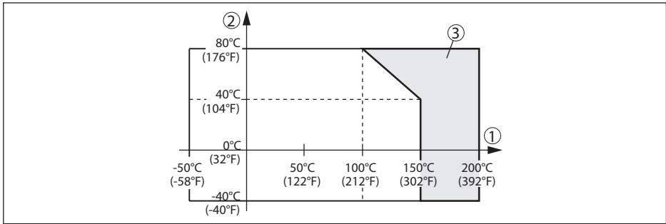
插图. 31: 环境温度 - 过程温度
