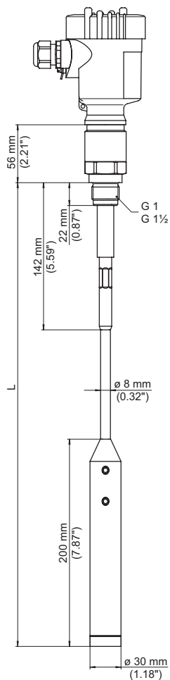
插图. 36: VEGACAL 65, 绳型 \varnothing 8 \text{ mm} (0.315 in), 螺纹型 G1 (ISO 228 T1)
