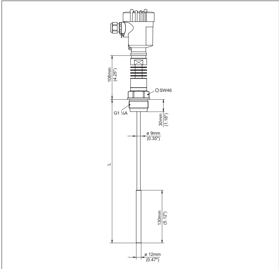
插图. 37: VEGACAL 65, PTFE 绝缘绳 (ø 8 mm) 带压接管 / -50 ... +200 °C
