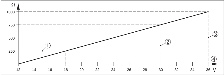
插图. 32: 供电电压图
