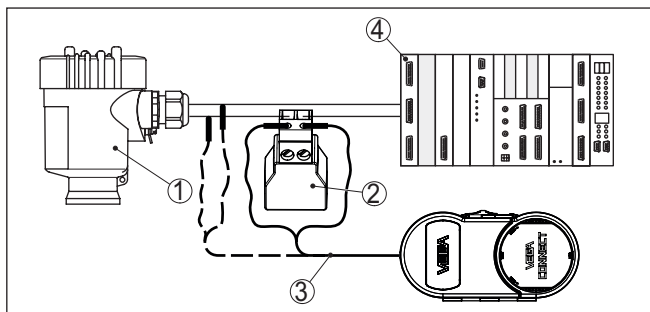
插图. 25: 通过 HART 将电脑与信号线路相连
