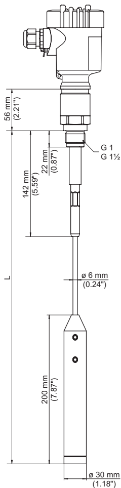
插图. 35: VEGACAL 65, 绳型 \varnothing 6 mm (0.236 in), 螺纹型 G1 (ISO 228 T1)
