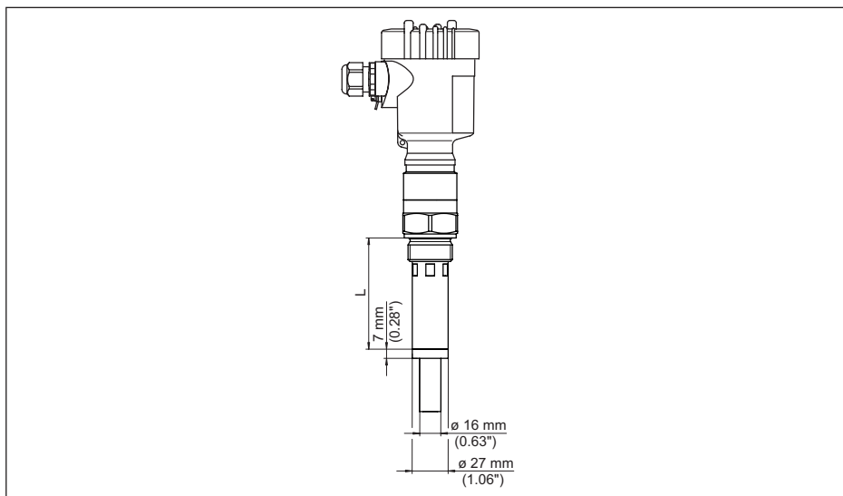
插图. 39: VEGACAL 65, 屏蔽管, 如用于防止冷凝水大量积聚
