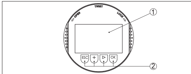
插图. 20: 显示和调整元件
