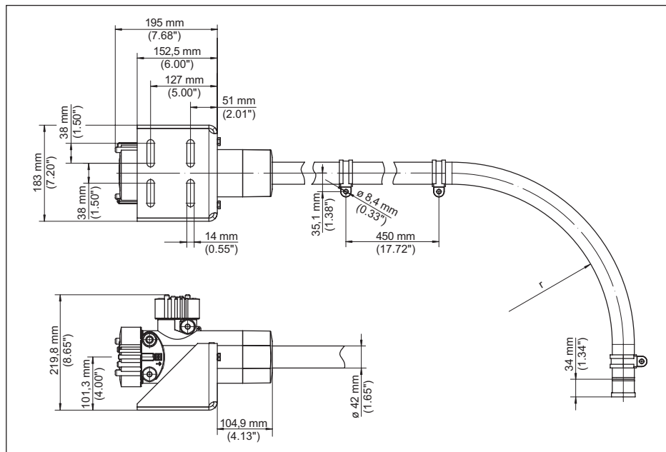
插图 31: FIBERTRAC 31 带随附的安装配件
