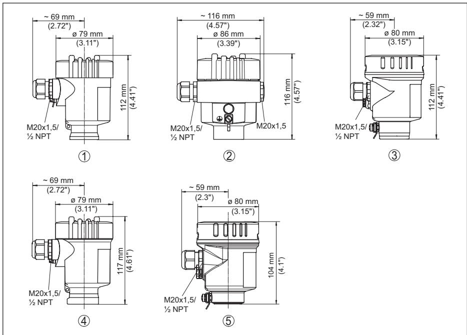
插图 28: 采用保护等级达 IP66/IP67 和 IP66/IP68 (0.2 bar) 的壳体版本。(内装显示和调整模块后，壳体高度增加了 9 mm/0.35 in 或 18 mm/0.71 in)
