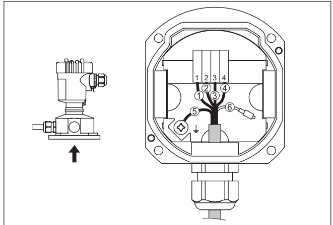
插图. 14: 壳体底座中过程组件的接口
