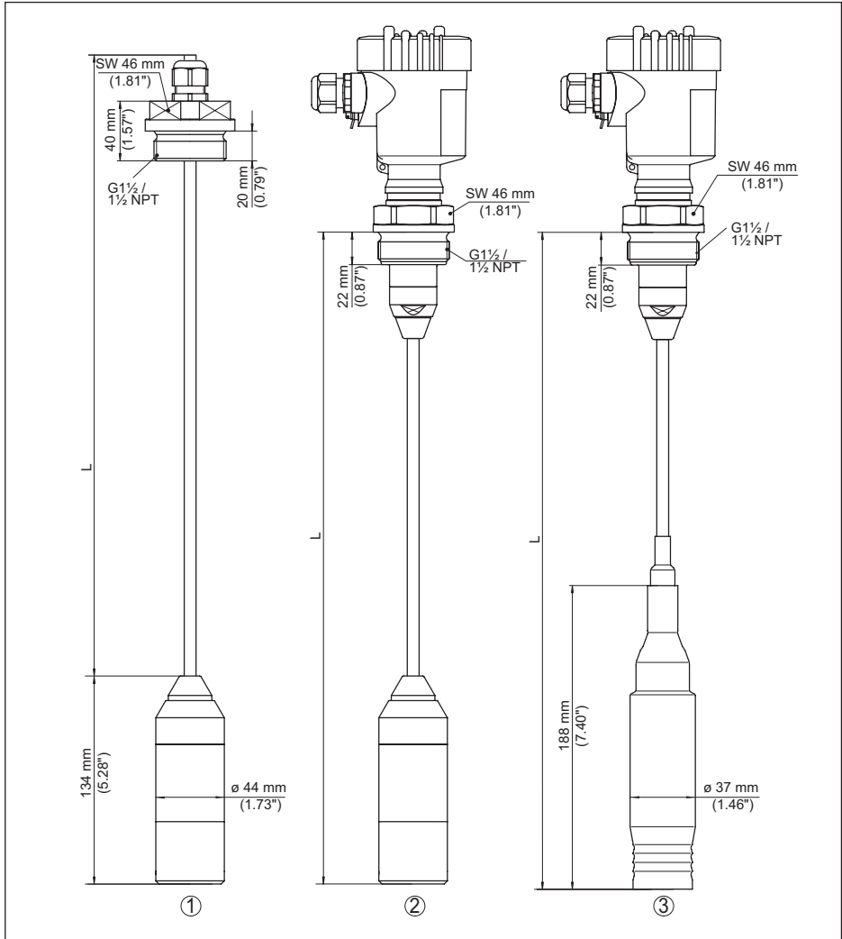
插图. 32: VEGABAR 86, 塑料型
