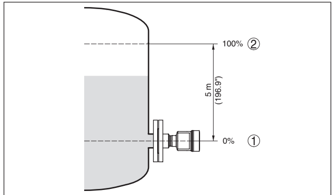
插图. 20: 物位测量时最小/最大调整的参数更改举例
