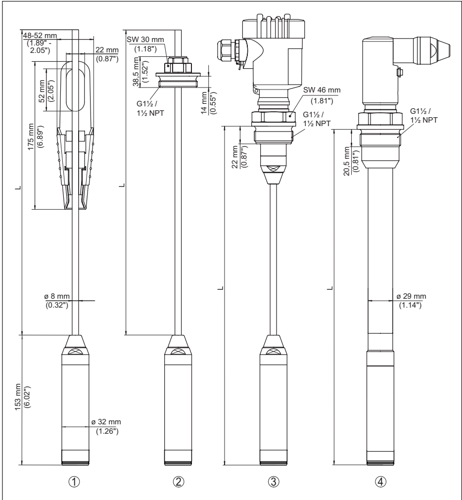
插图. 30: VEGABAR 86, 测量值记录仪 (32 mm)
