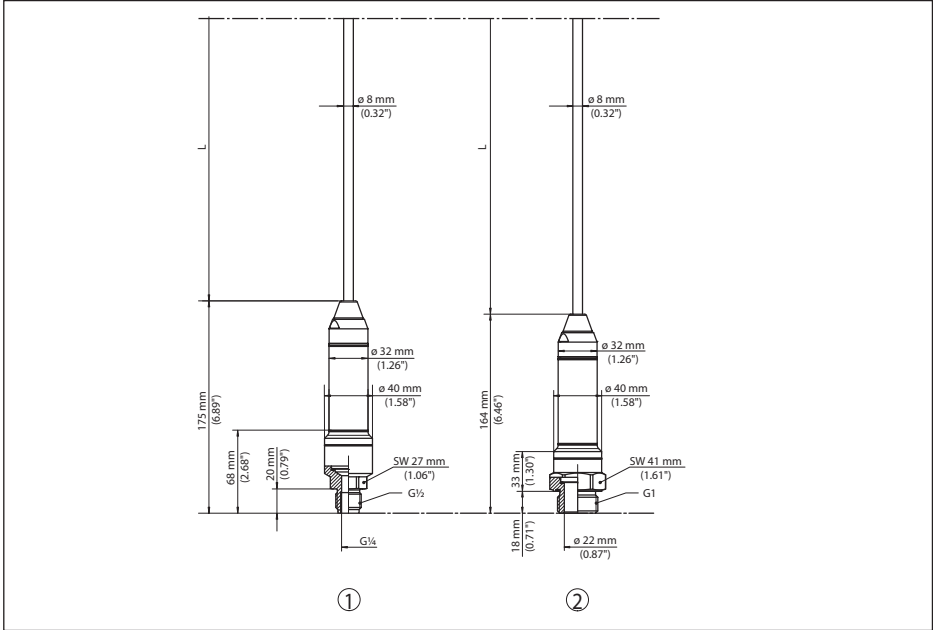
插图. 35: VEGABAR 86, 螺纹型
