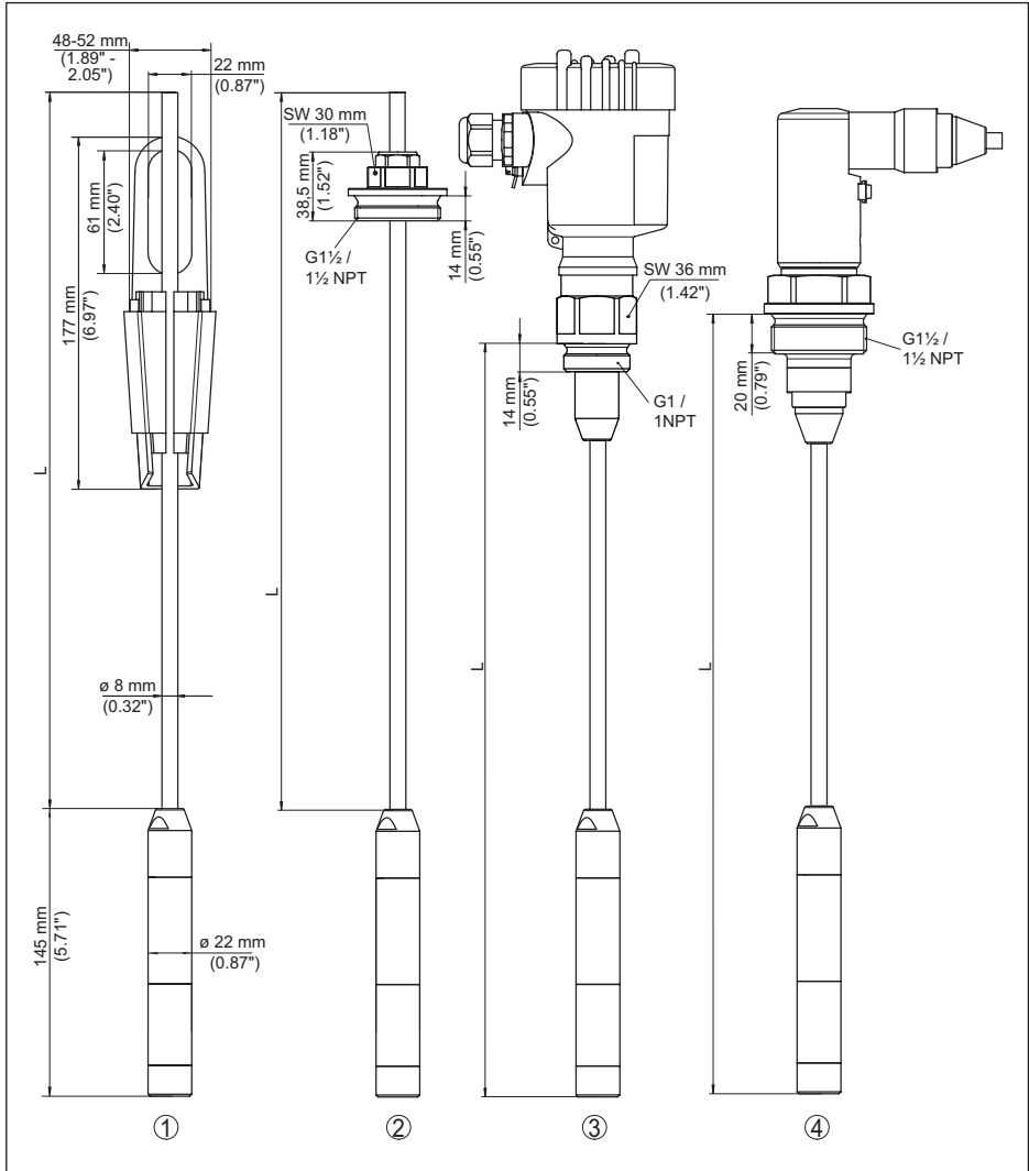
插图. 31: VEGABAR 86, 测量值记录仪 (22 mm)
