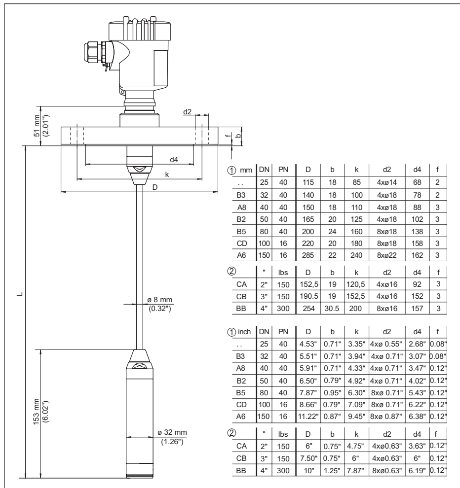
插图. 33: VEGABAR 86, 法兰连接 (用 32 mm 测量值记录仪为例说明)
