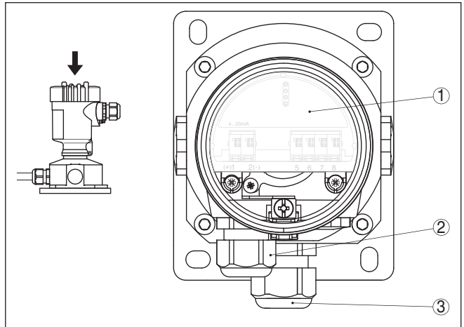
插图. 15: 电子部件腔和接线腔
