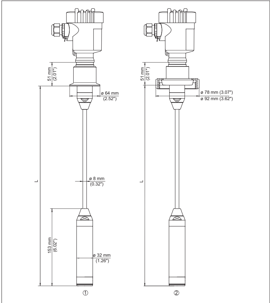
插图. 34: VEGABAR 86, 无菌接口
