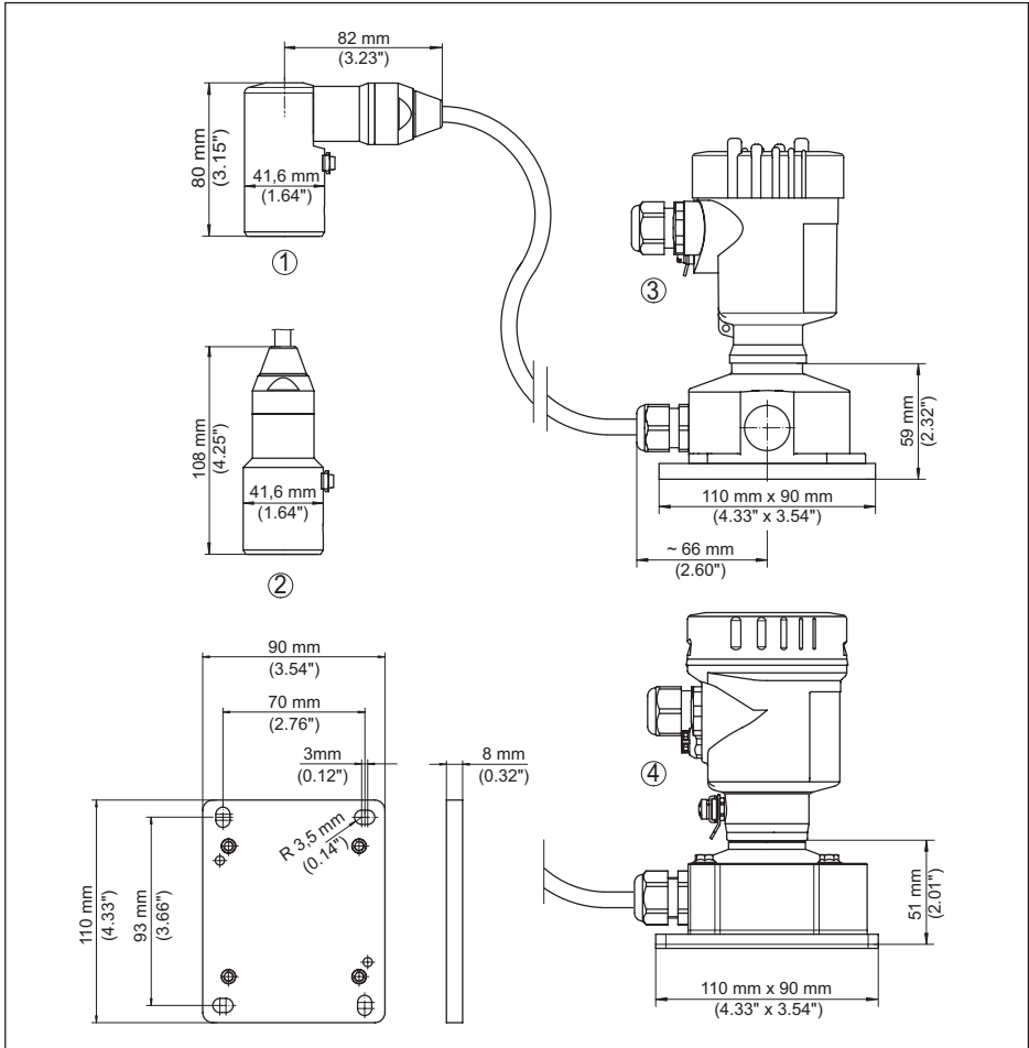
插图. 29: VEGABAR 86, IP68 型, 带外部壳体
